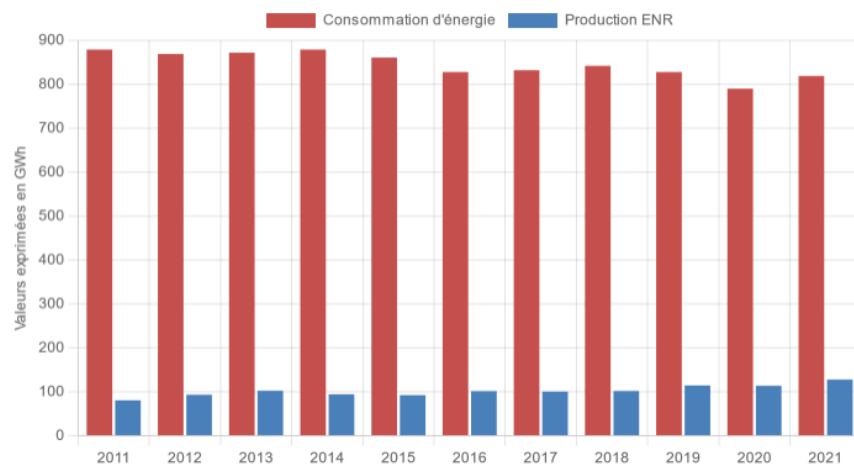
Evolution comparée de la consommation d'énergie finale et de la production d'énergie renouvelable locale
