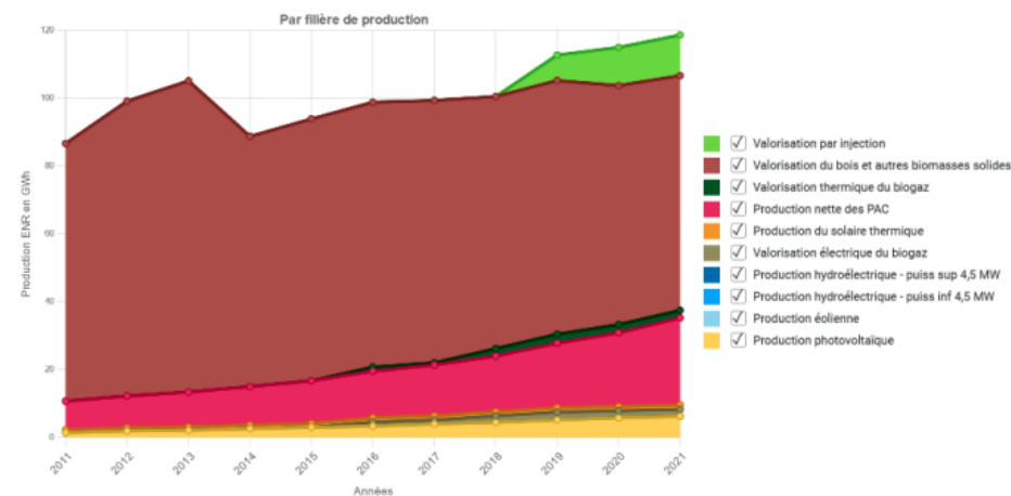
Évolution de la production EnR (en GWh)
